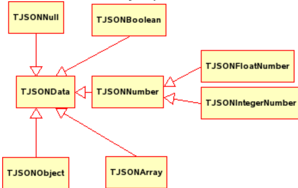
Figure 3: jsondata
